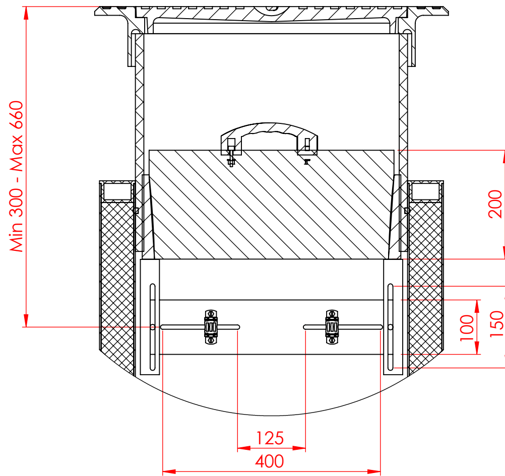
Detalizācija C Mērogs 1 : 7
