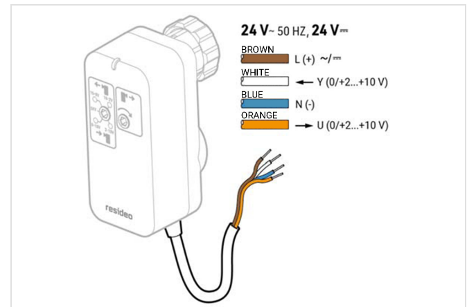
Fig. 5 Electrical wiring
